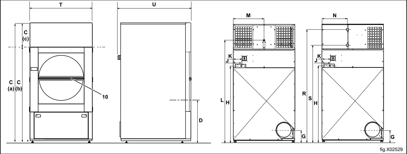
10 | Abertura de la puerta con puerta deslizante, ø 940 mm
